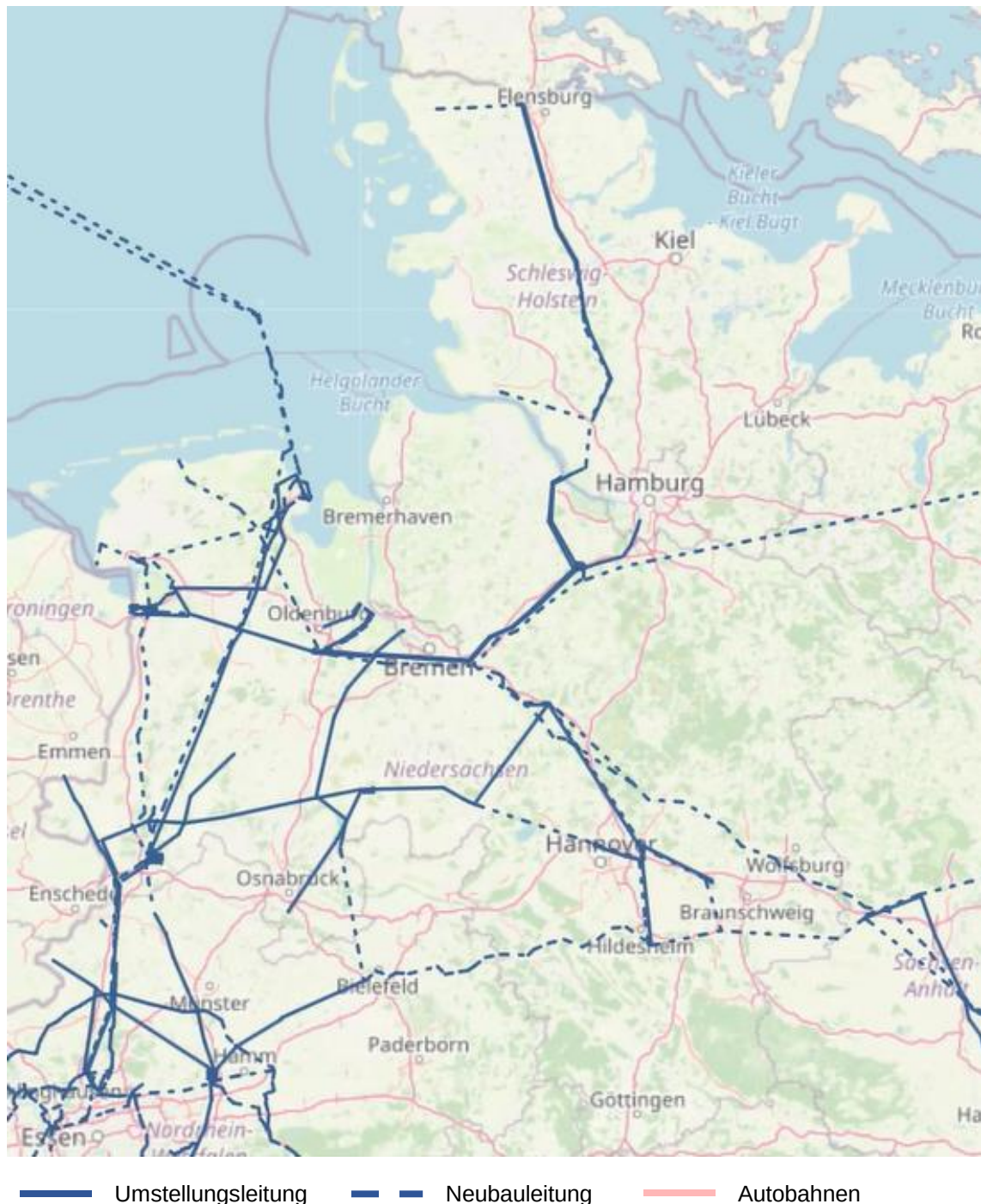
Abbildung 5: Aktueller Planungsstand des Wasserstoff-Kernnetzes in der Region Nordwest
