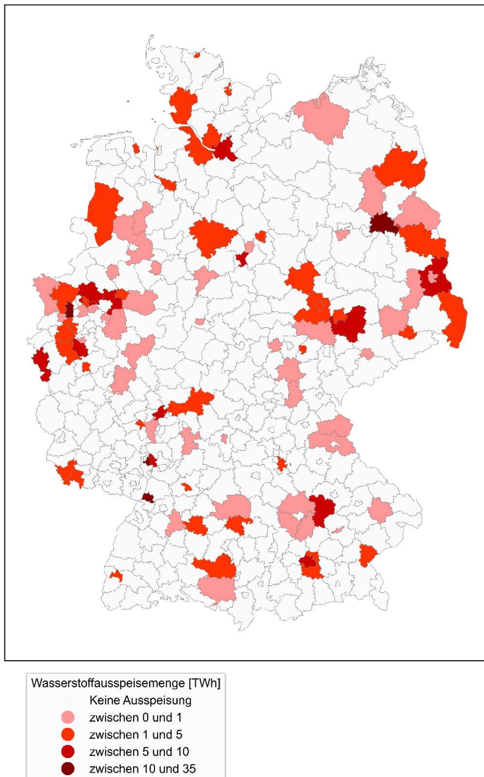
Abbildung 2: Ausspeisemengen für Wasserstoff auf Kreisebene im Szenario für das Wasserstoff-Kernnetz, Angaben für das Jahr 2032 in TWh als Brennwert
